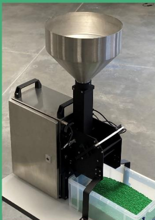
SPECTRO-T-3-0°/45°-LAB-LF SPECTRO-T-3-DIF/0°-LAB-LF
